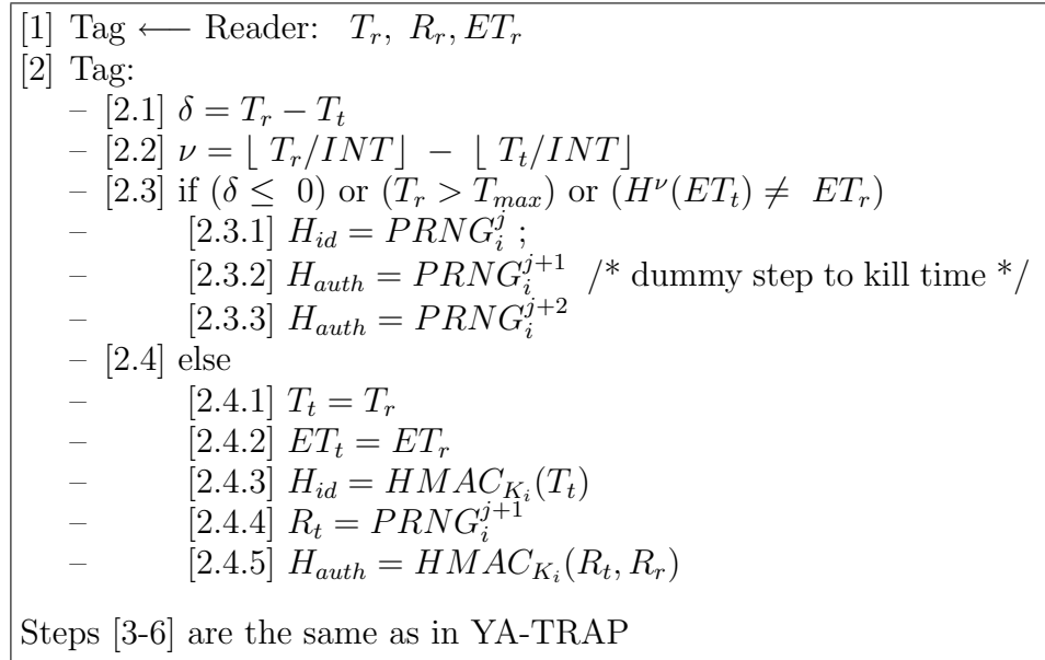
Fig. 3. YA-TRAP*: DoS Resistance
